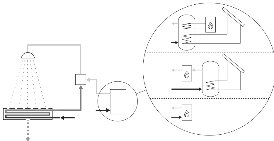
C Anschluss an Warmwasserbereitung / Connection to DHW generator / Raccord au chauffe-eau / Aansluiting op de boiler
